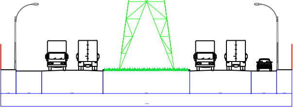
SECCIÓN X - X (Servidumbre de línea eléctrica de 220 kV)
