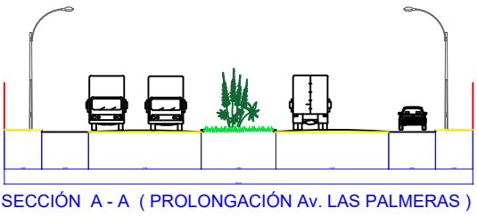
SECCIÓN A - A ( PROLONGACIÓN Av. LAS PALMERAS )
